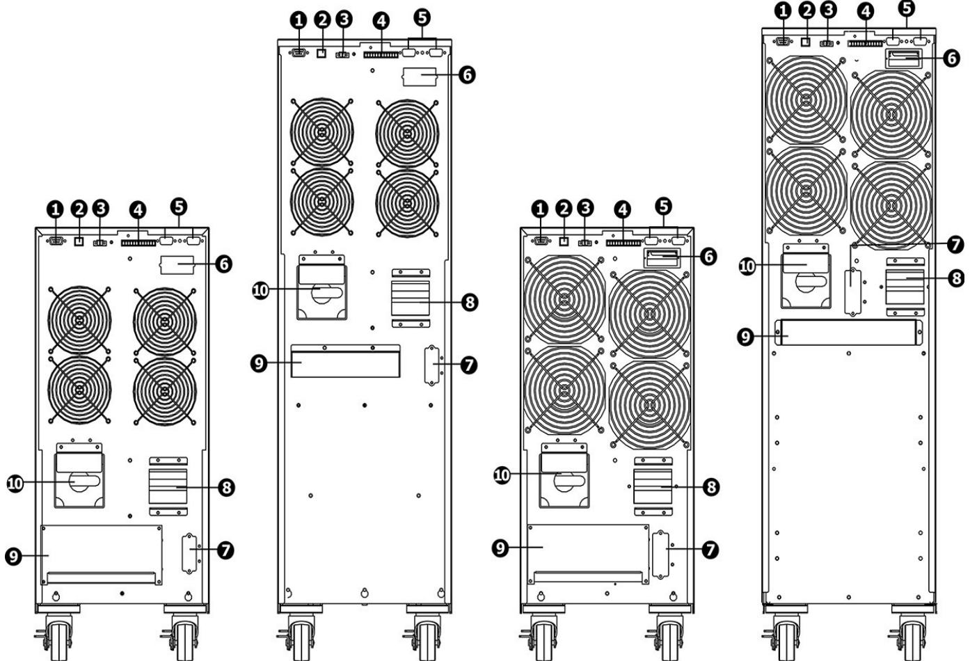
Рис.2-2 Внешний вид задней панели ИБП.
